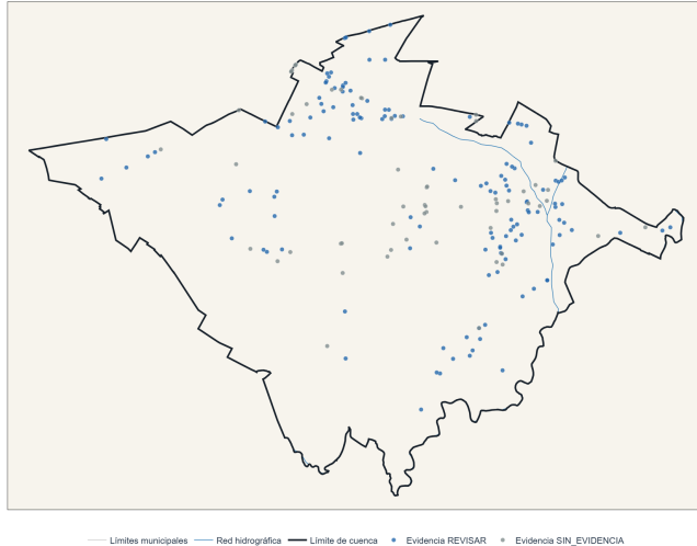
San Andrés Cholula: establecimientos con potencial hídrico
